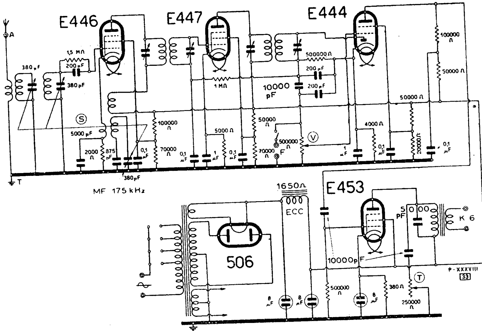
WATT RADIO - MOD. « APOLLO »
